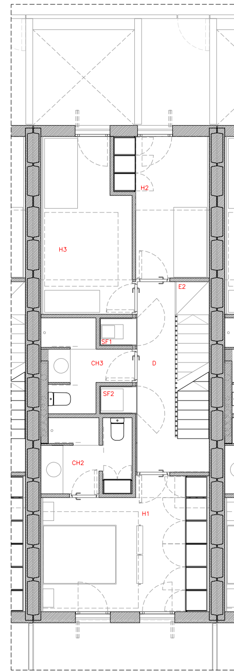
HABITATGE TIPUS 1A - PLANTA PRIMERA E 1:100
