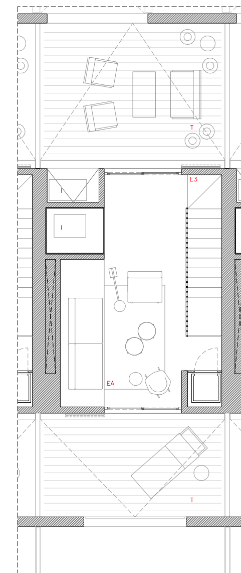
HABITATGE TIPUS 1 - PLANTA COBERTA E 1:100
