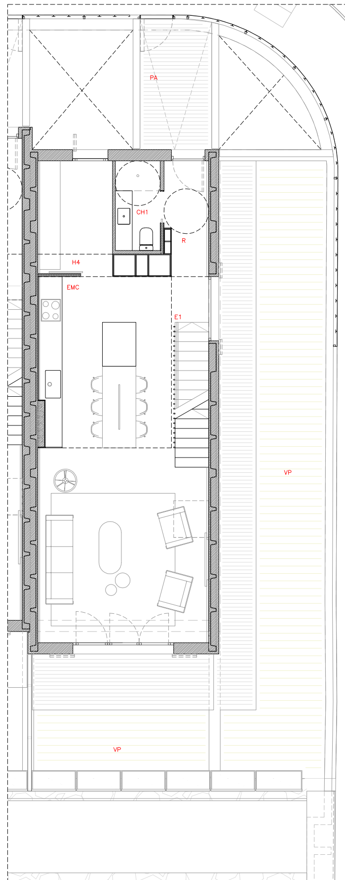
HABITATGE TIPUS 1C - PLANTA BAIXA E 1:100
