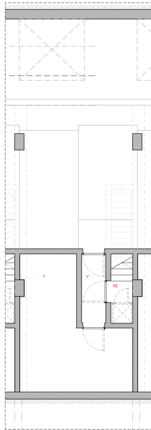
HABITATGE TIPUS 1A - PLANTA SOTERRANI E 1:100
