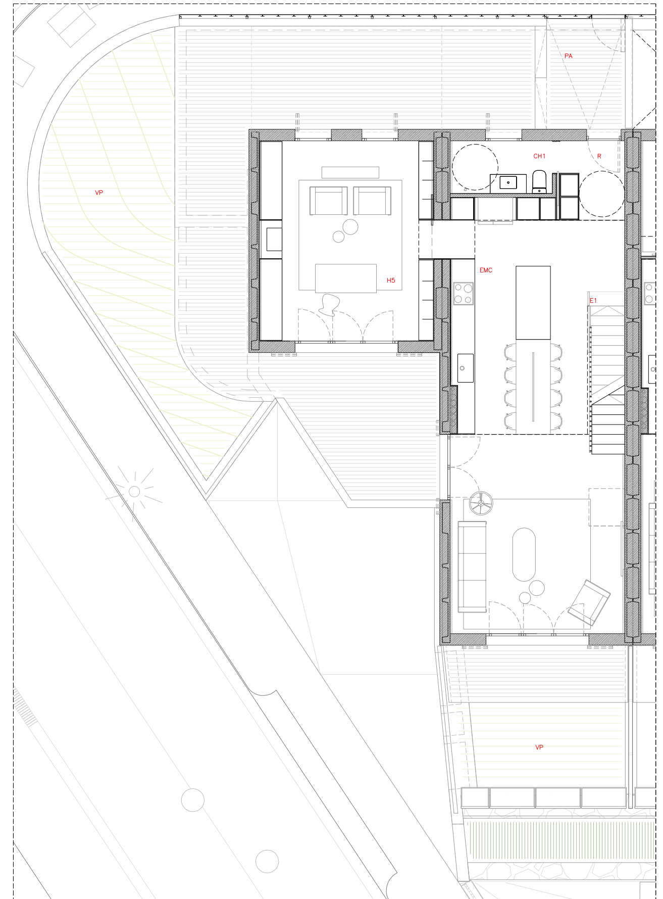
HABITATGE TIPUS 2 - PLANTA BAIXA E 1:100
