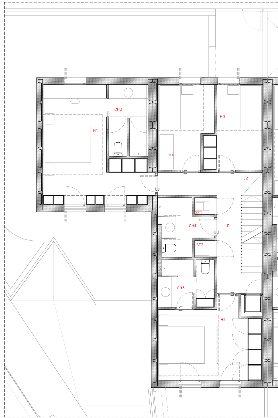
HABITATGE TIPUS 2 - PLANTA PRIMERA E 1:100
