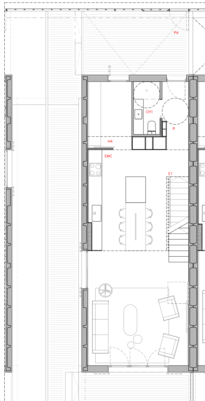
HABITATGE TIPUS 1B —PLANTA BAIXA E 1:100
