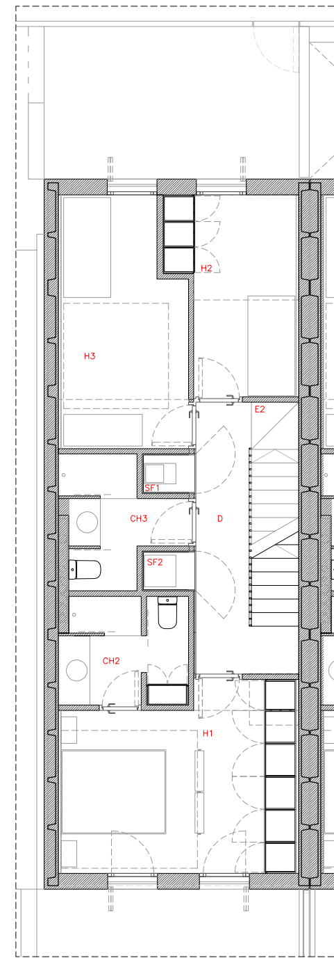
HABITATGE TIPUS 1B—PLANTA PRIMERA E 1:100
