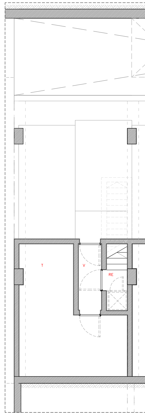
HABITATGE TIPUS 1B—PLANTA SOTERRANI E 1:100
