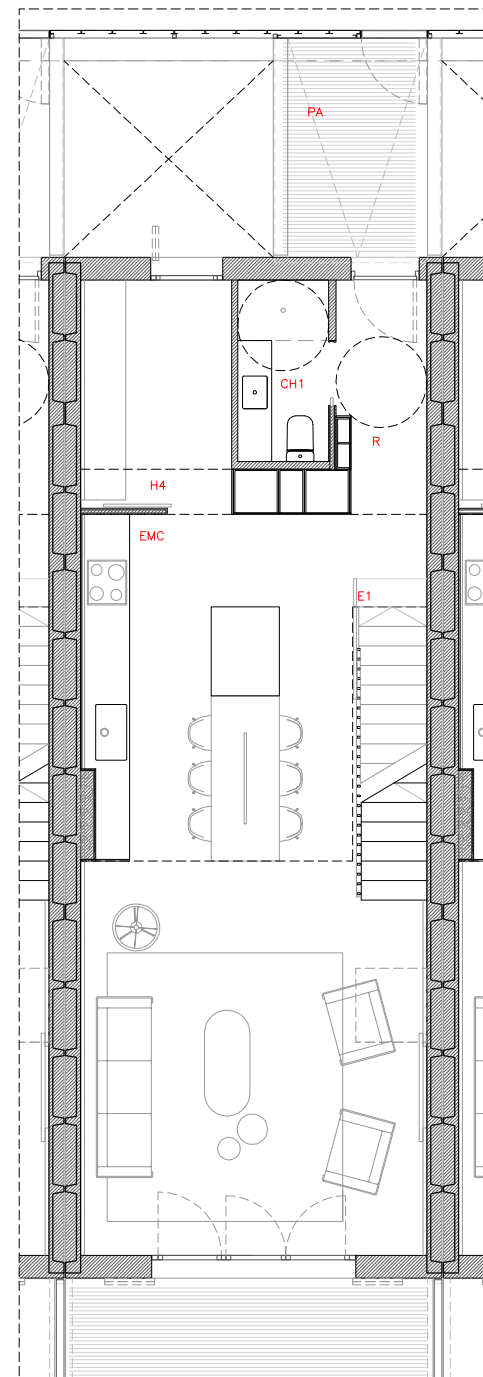
HABITATGE TIPUS 1A - PLANTA BAIXA E 1:100
