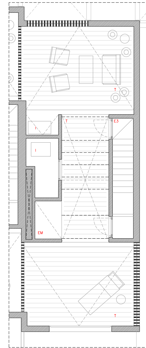
HABITATGE TIPUS 1C - PLANTA COBERTA E 1:100
