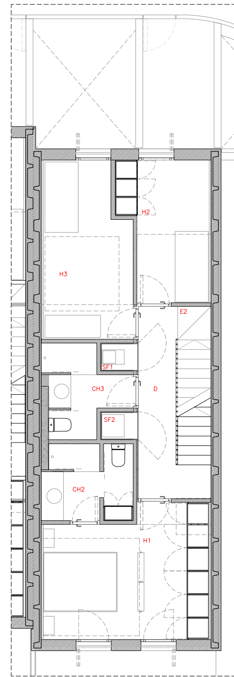
HABITATGE TIPUS 1C - PLANTA PRIMERA E 1:100
