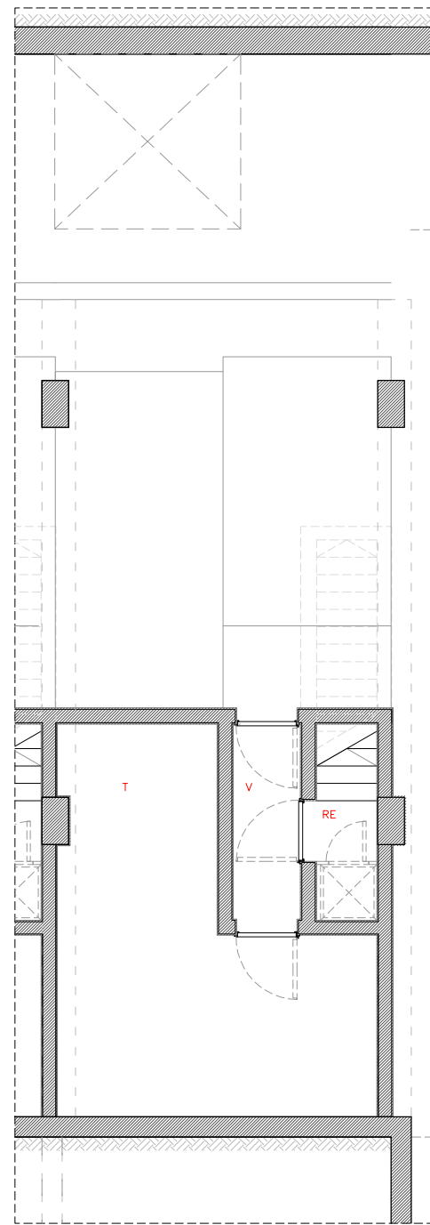
HABITATGE TIPUS 1D - PLANTA SOTERRANI E 1:100
