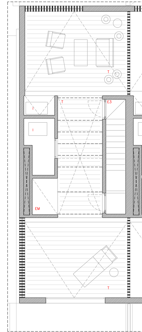
HABITATGE TIPUS 1B —PLANTA COBERTA E 1:100
