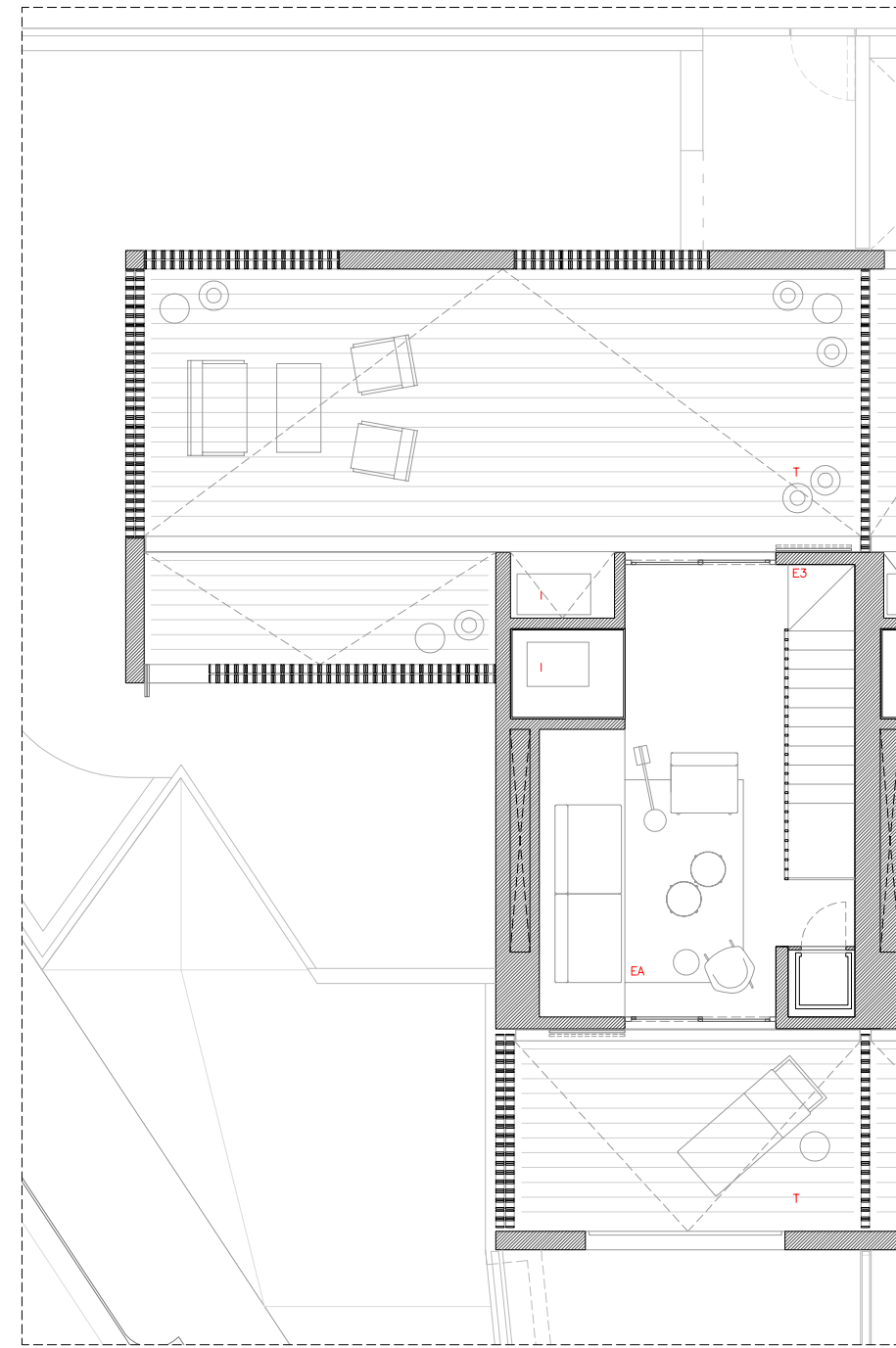
HABITATGE TIPUS 2 - PLANTA COBERTA E 1:100
