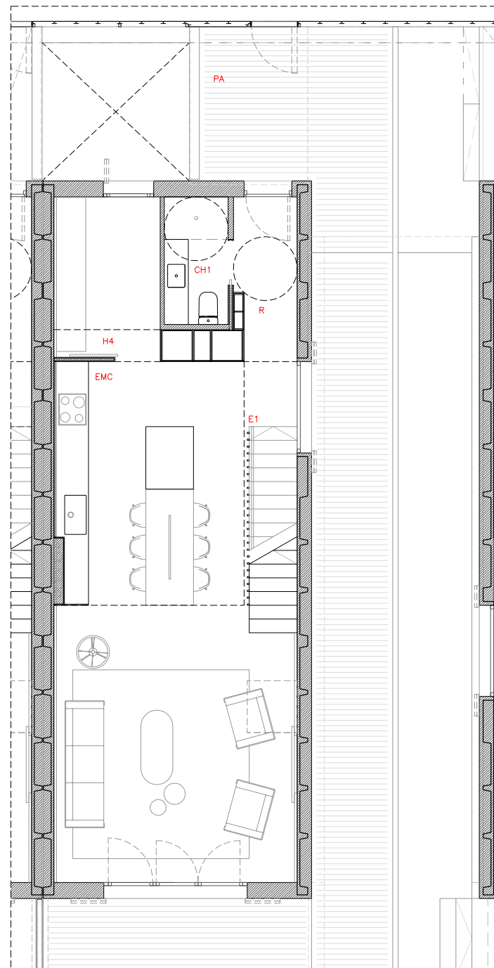
HABITATGE TIPUS 1D - PLANTA BAIXA E 1:100
