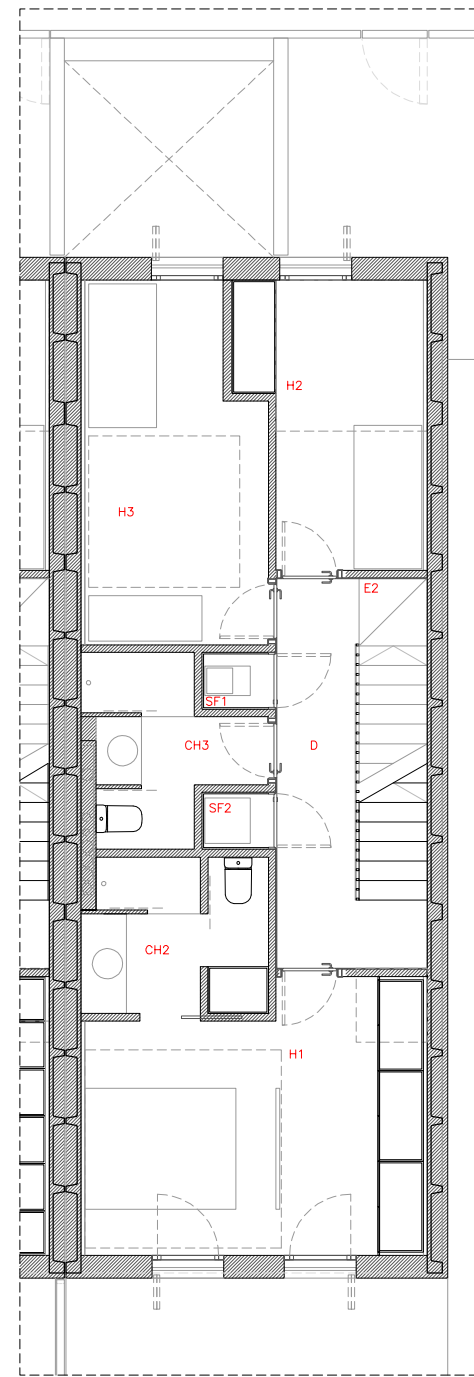
HABITATGE TIPUS 1D - PLANTA PRIMERA E 1:100
