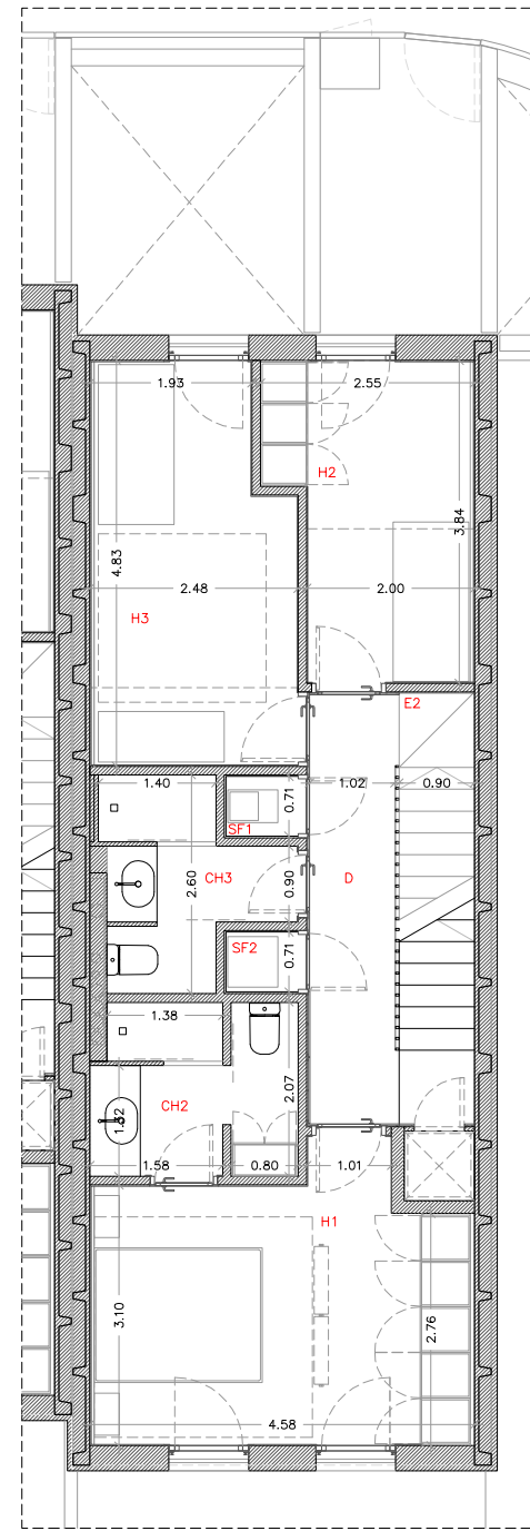
HABITATGE TIPUS 1 - PLANTA BAIXA E 1:100
